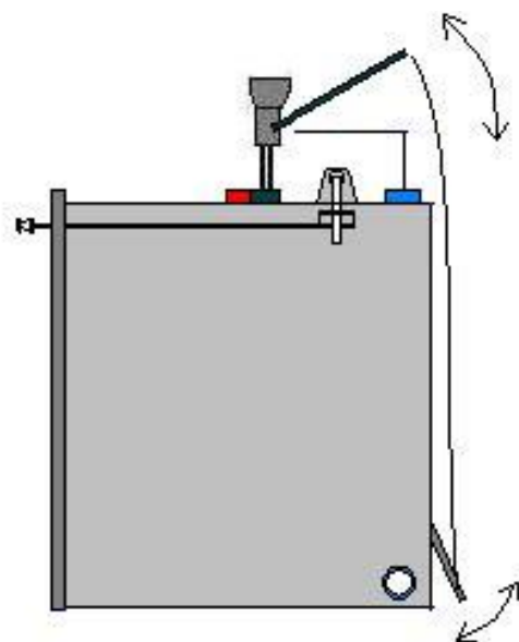
Figura 4. Esquema de montagem do regulador de combustão
