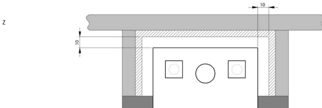
Figura 3. Revestimento do espaço de inserção – paredes combustíveis e isolamento
